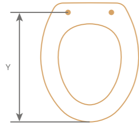
PROFONDITÀ | DEPTH Dai fori alla punta From holes to the tip
